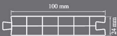
پنل لامبری LAMBRY PANEL PROFILE ▶
