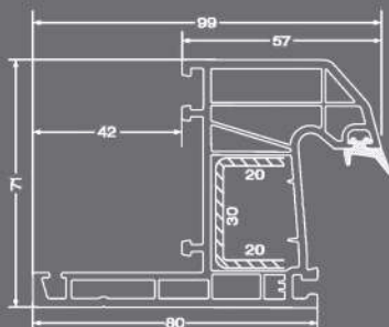
پروفیل قاب بازسازی RENOVATION FRAME PROFILE
