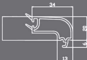
زهوار شیشه تک جداره SINGLE GLASS GLAZING BEAD ▶
