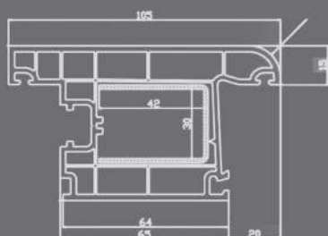
پروفیل لنگه بیرون بازشو درب OUT DOOR SASH PROFILE ▶
