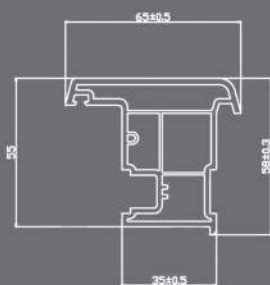
پروفیل میانی متحرک FALSE MULLION PROFILE ▶
