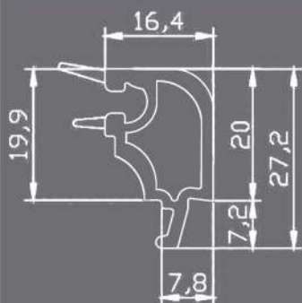
زهوار شیشه دوجداره DOUBLE GLASS GLAZING BEAD
