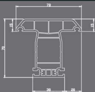
پروفیل میانی ثابت MULLION PROFILE
