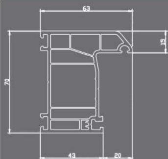
پروفیل لنگه داخل بازشو درب IN DOOR SASH PROFILE ▶
