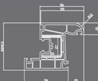
پروفیل لنگه پنجره SASH PROFILE ▶
